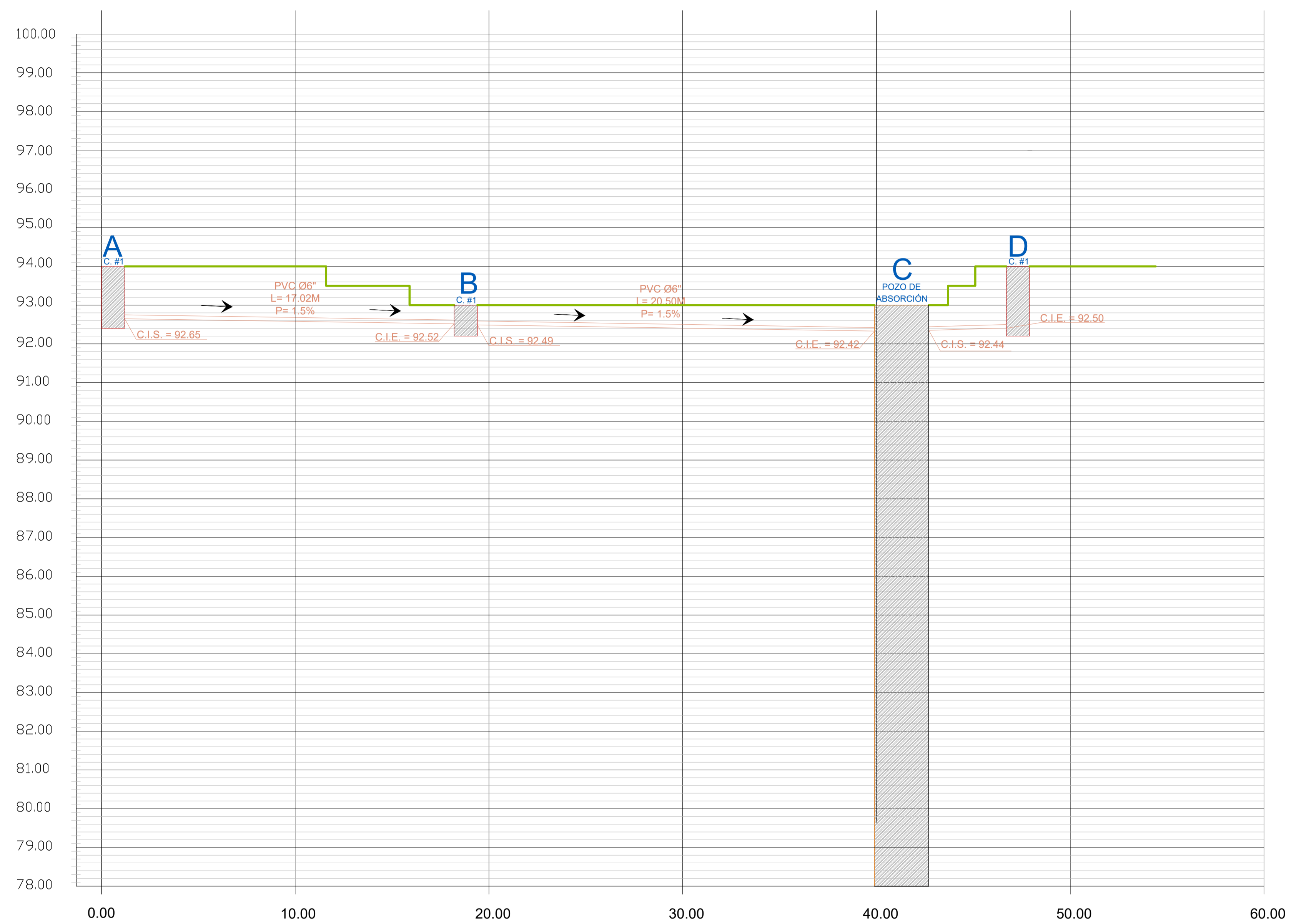
PERFIL DRENAJE PLUVIAL PERFIL ESCALA HORIZONTAL 1:150 ESCALA VERTICAL 1:75
